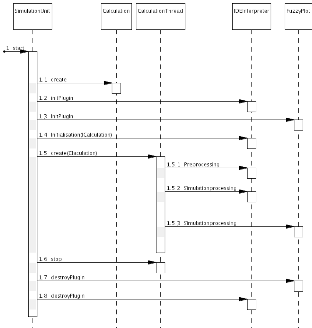
Abbildung 12.7.: Sequenzdiagramm Simulator
