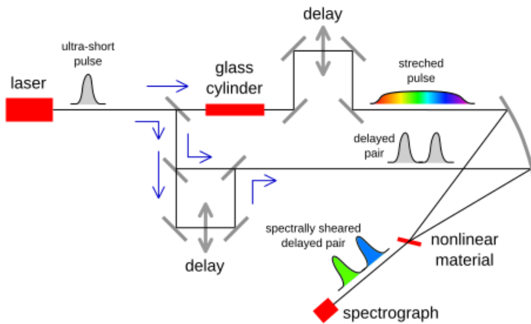
Figure 1.4: * Schematischer Versuchsaufbau für SD-SPIDER.
